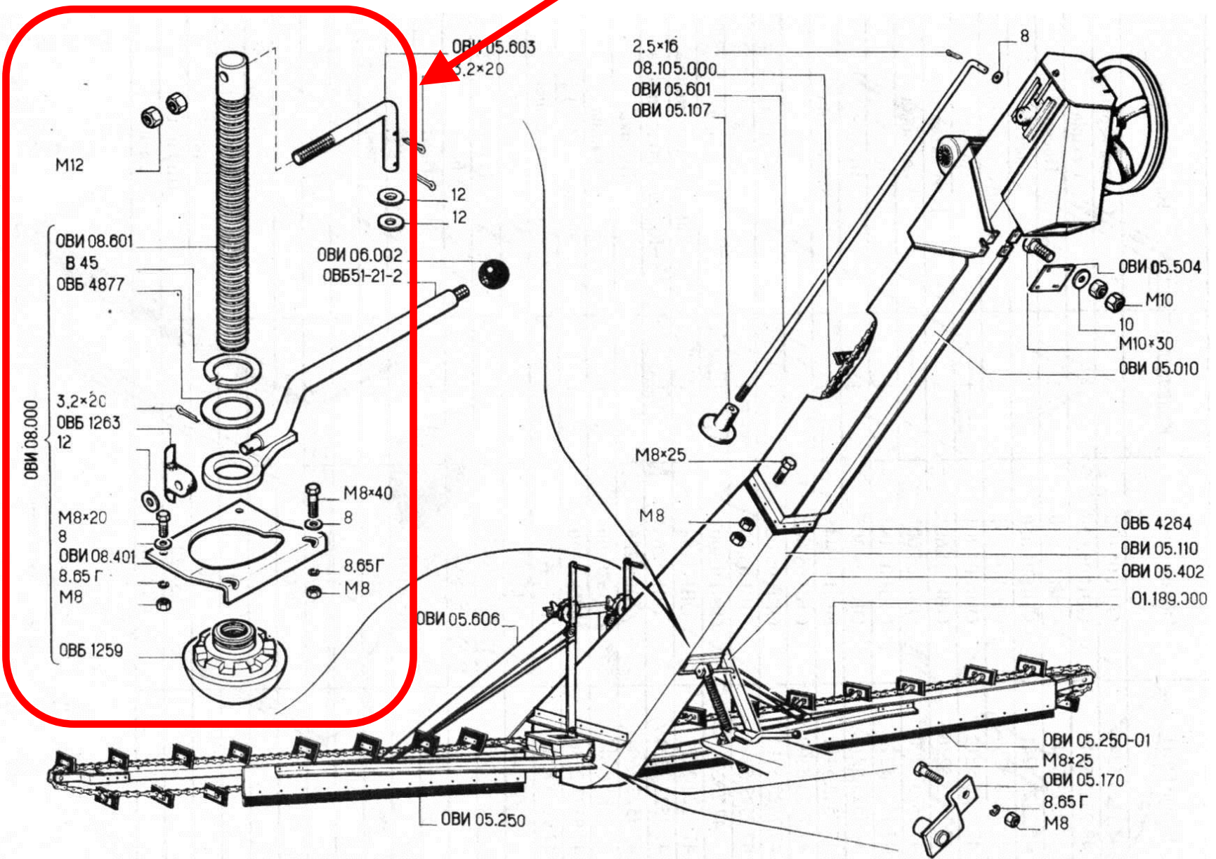
Рис. 23. Транспортёр загрузочный ОВИ 05.000.
