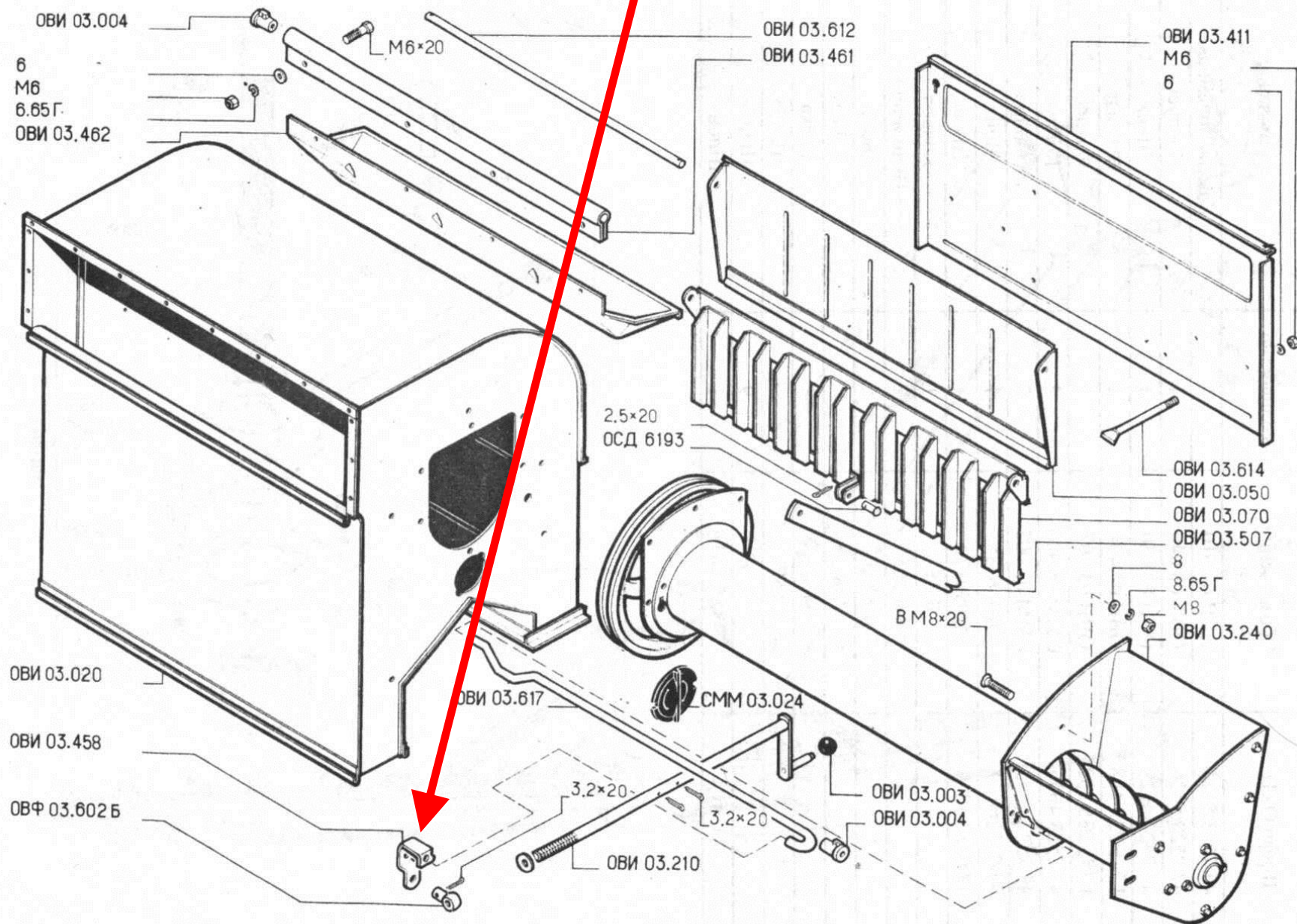
Рис. 16. Камера приемная ОВИ 03.010.
