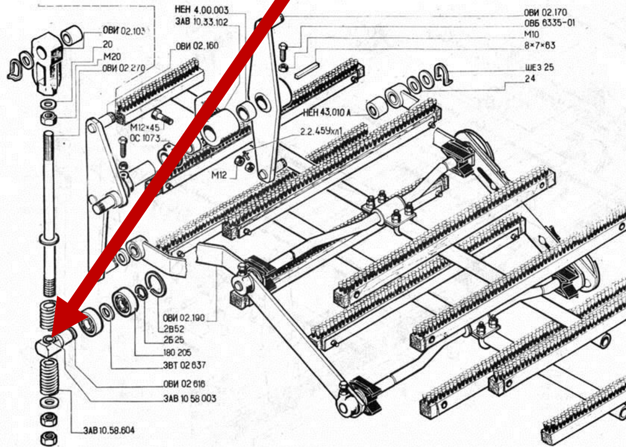
Рис. 12. Механизм очистки решет. ОВИ 02.150.
